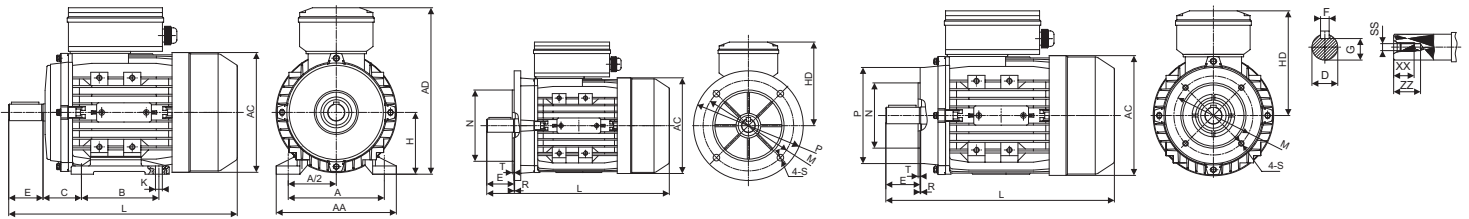
IM B3
