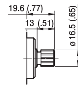
DIN 5482 B17x14
