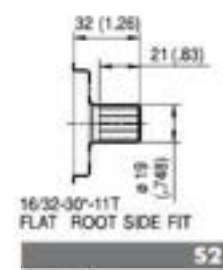
S2 Coppia Max Max Torque 230 Nm
