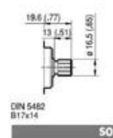
SO Coppia Max Max Torque 130 Nm
