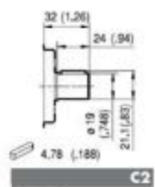
C2 Coppia Max Max Torque 150 Nm
